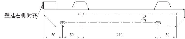
图 4.7 壁挂架规格图
