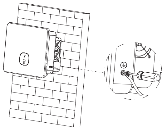
图 5.1 接地示意图
