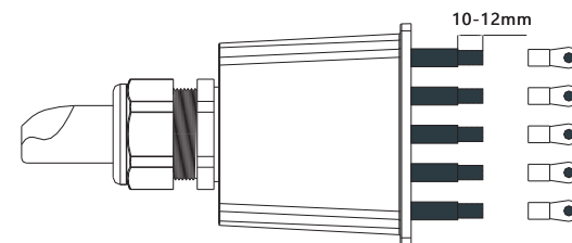
图 5.2 AC输出线压接端子示意
