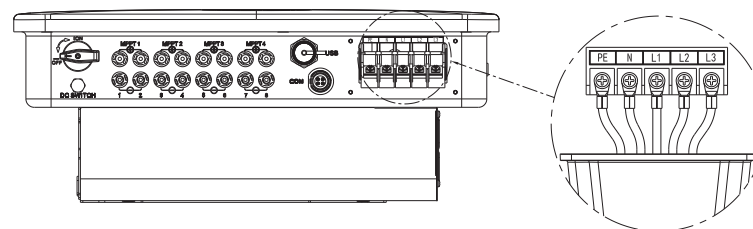
图 5.3 AC端子接线示意
