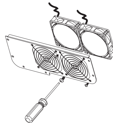
图 11.2 拆风扇示意
