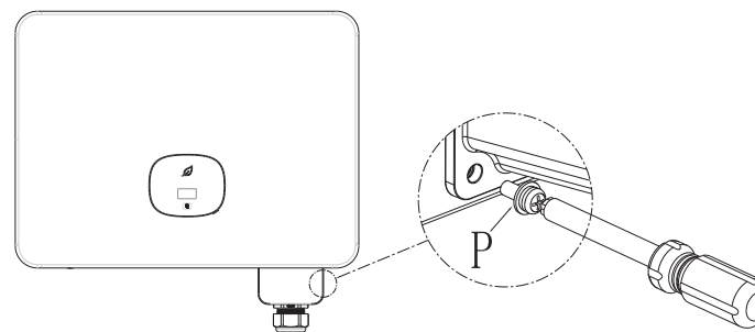
图 5.4 AC端锁防水罩示意
