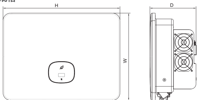
图 2.2 尺寸规格
