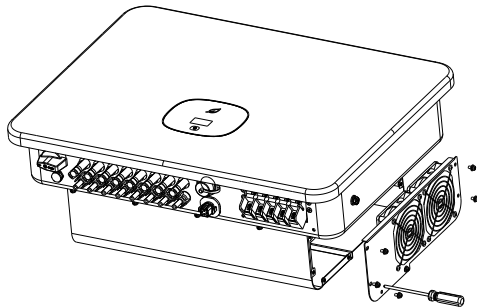
图 11.1 拆风扇固定板示意
