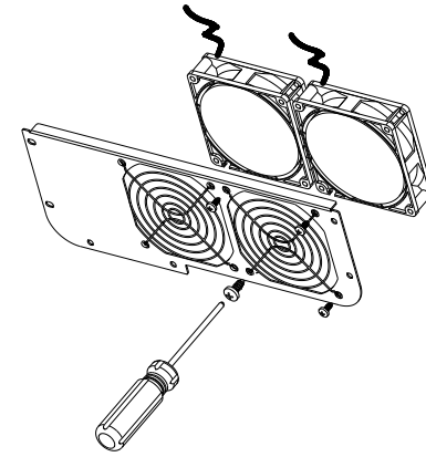
图 11.2 拆风扇示意
