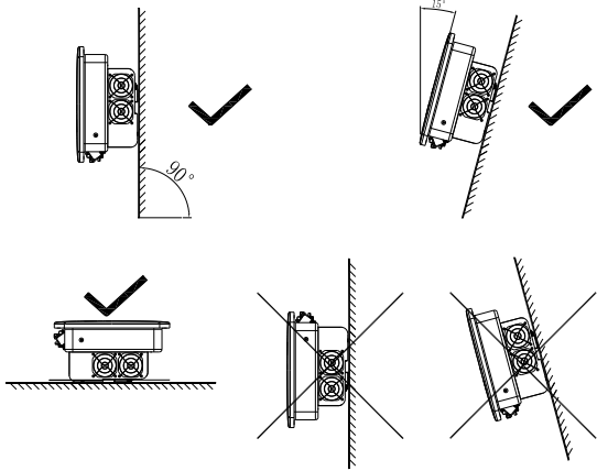
图 4.1 安装示意图
