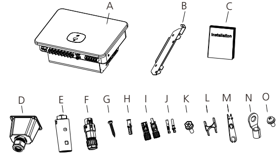
图 3.1 配件图
