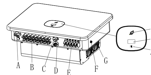
图 2.1 外观概图
