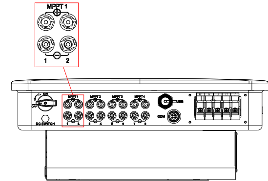
图 5.5 PV端子
