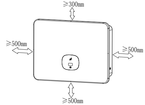
图 4.2 一台逆变器时的安装尺寸
