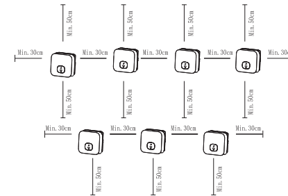
图4.3 多台逆变器时的安装尺寸
